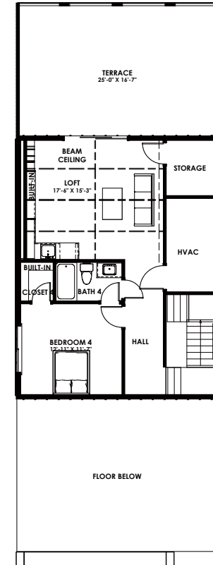
LOFT
